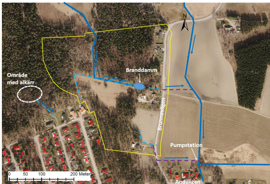
Figur 2. Planområde (gul linje), diken som ingår i markavvattningsföretag (blå heldragna linjer), övriga öppna diken (blå streckade linjer), ungefärligt läge på kulvertar (lila linjer) samt läge för pumpstation.
